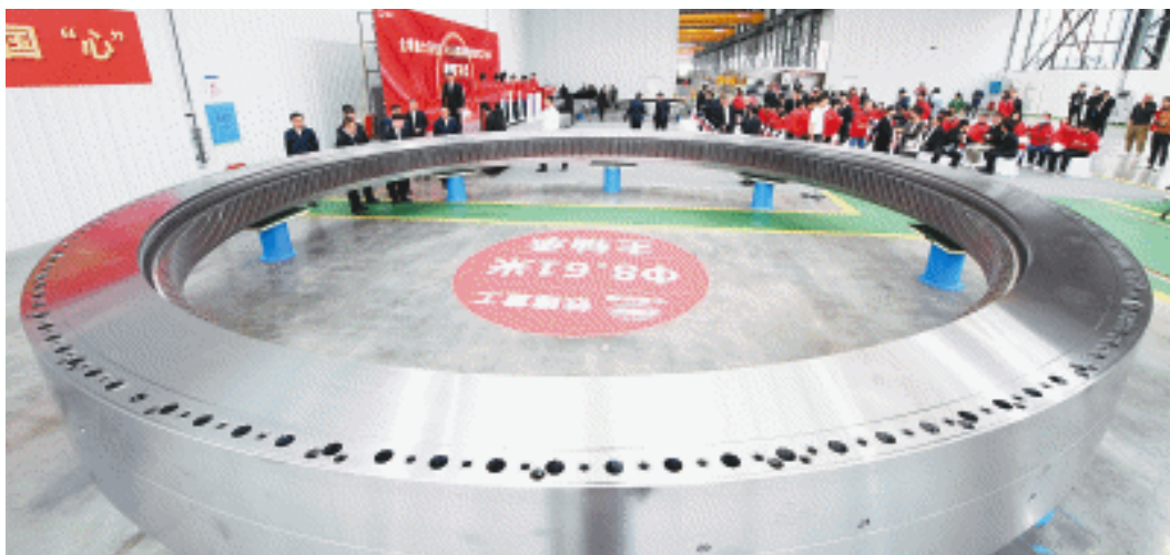
铁建重工自主研发的全球直径最大、单体最重、承载最高的整体式盾构机主轴承。王志伟 摄
